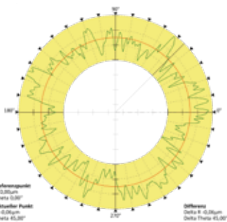
Rundheit vor Microfinish
